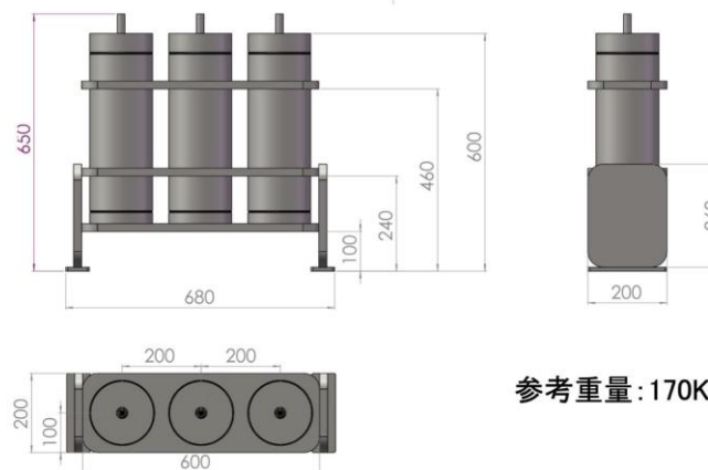
吸蔵合金タンク3本組参考図
